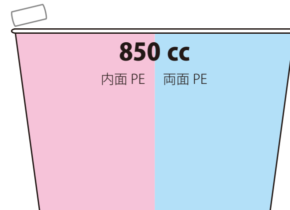
T 138φ(B 111φ)H88 FC890ml 25(PE)×20 : 500 Min lot 5,000～
